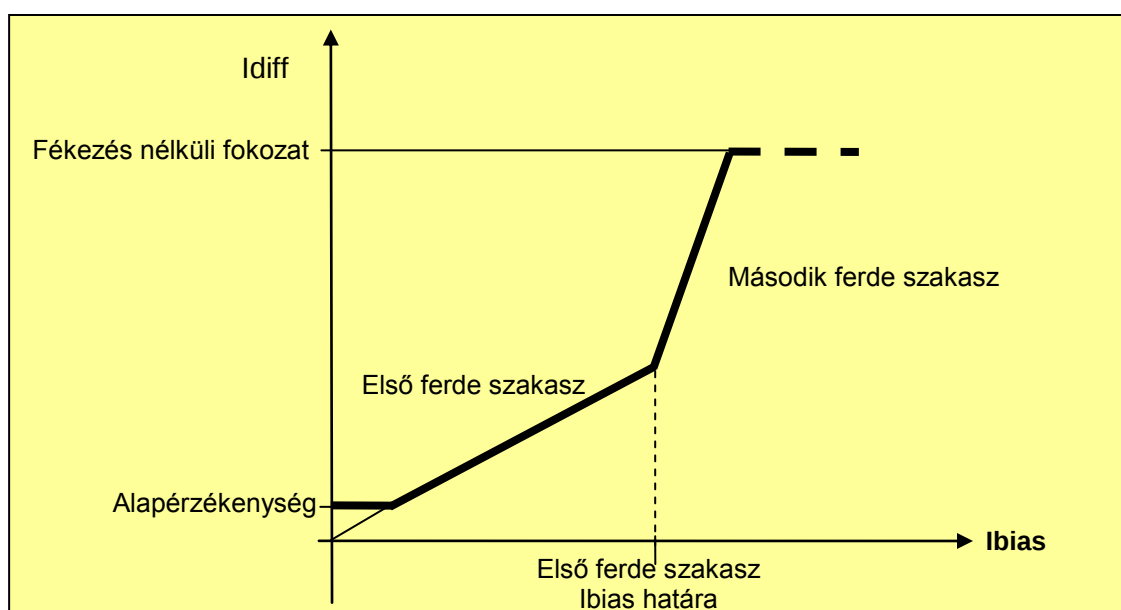
7. ábra Differenciál-karakterisztika
