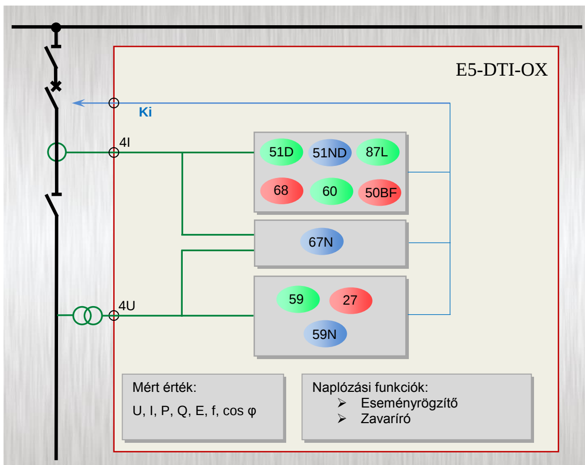
1. ábra Védelmi funkciók
