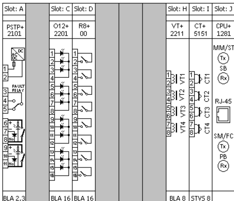
2. ábra Az E5-DTI-OX alap konfiguráció kártyakiosztása 42TE esetén (hátnézet)
