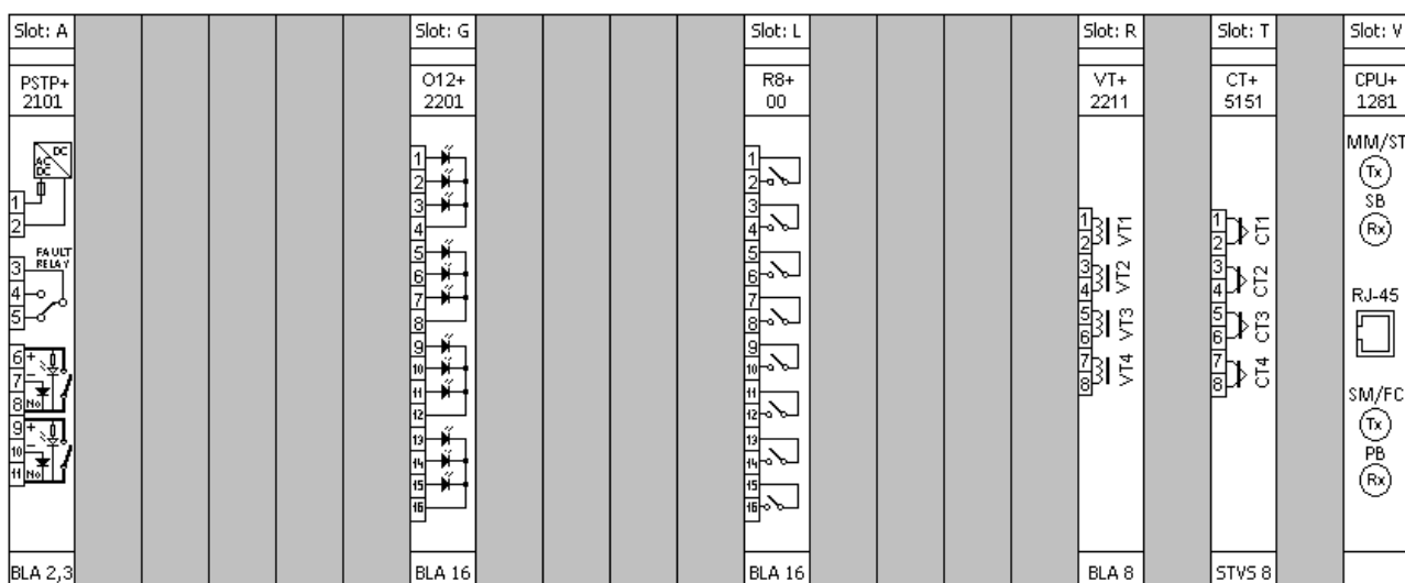
3. ábra Az E5-DTI-OX alap konfiguráció kártyakiosztása 84TE esetén (hátnézet)
