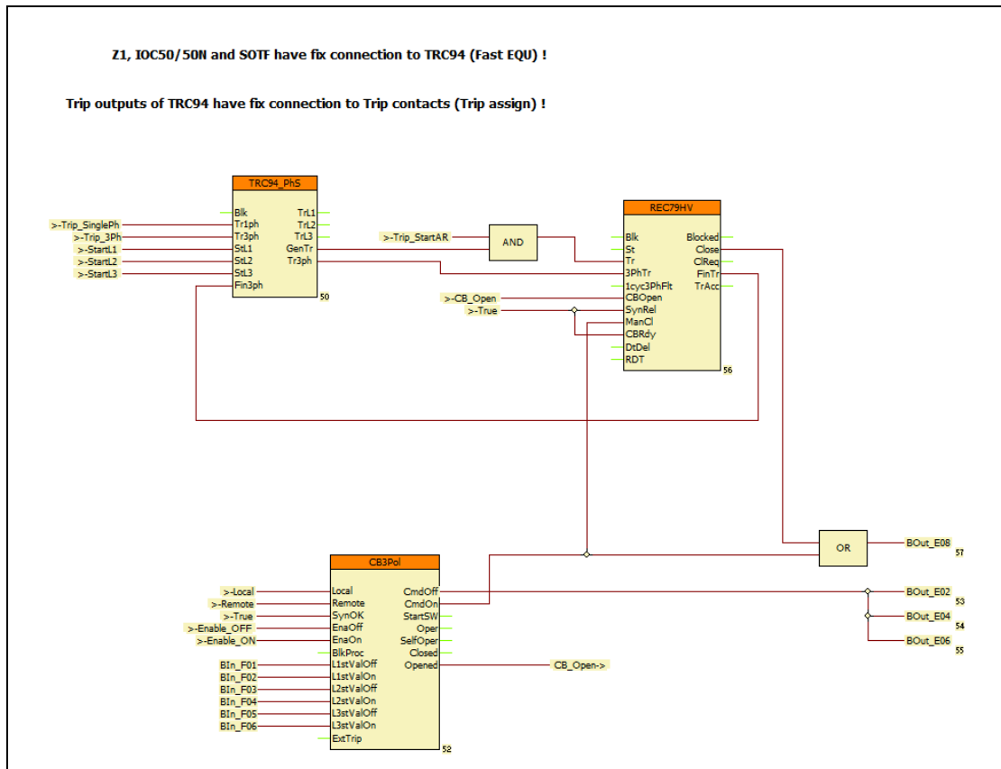
5-3. ábra Automatikus visszkapcsolás és megszakító vezérlés
